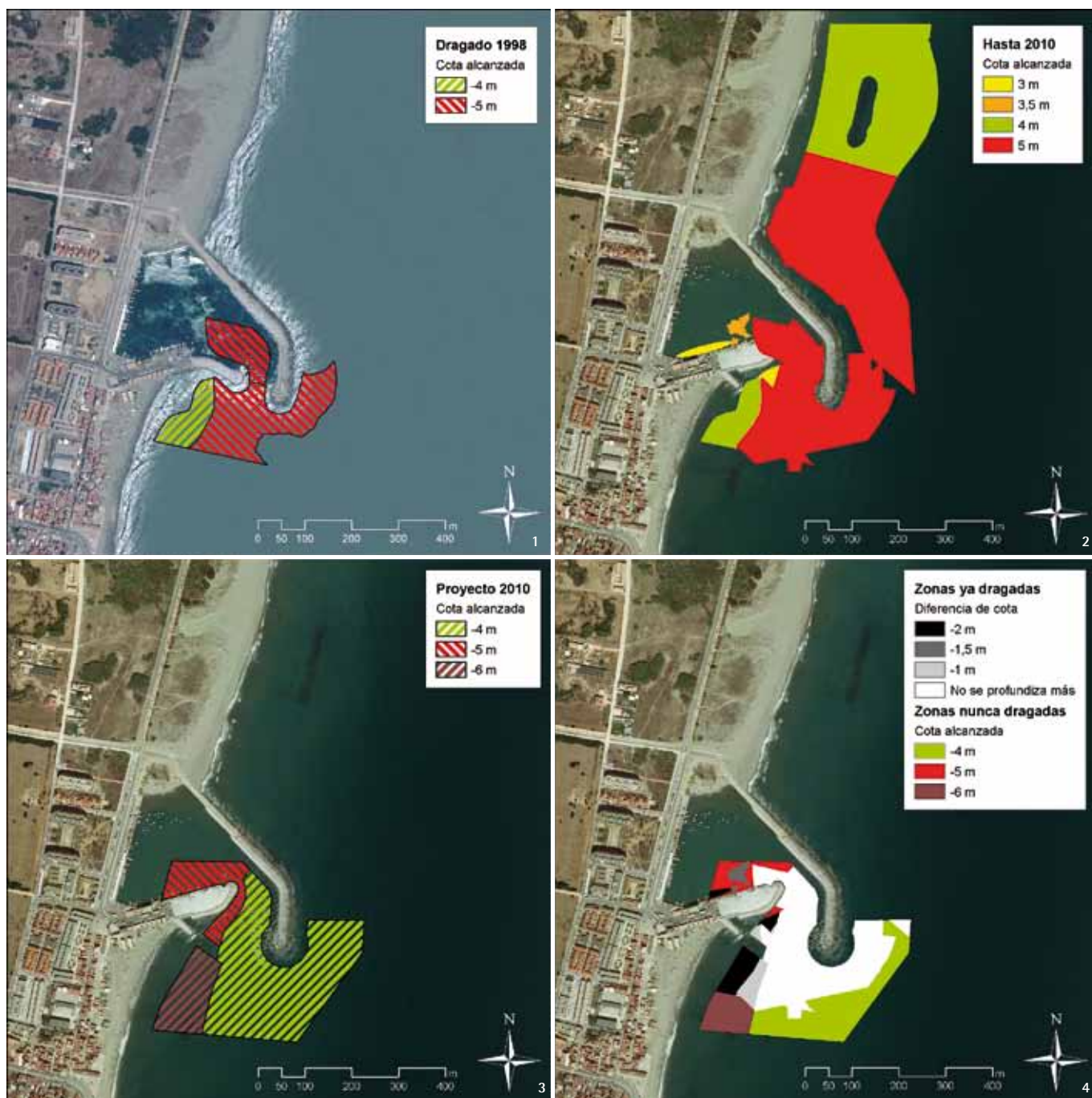
Aplicación de los SIG para el control de las obras de dragado. 1. Profundidades alcanzadas en el primer dragado realizado en 1998; 2. Profundidades máximas alcanzadas hasta el año 2010; 3. Profundidades que se pretende alcanzar en el proyecto de 2010; 4. Zonificación del proyecto 2010 en zonas ya dragadas y nunca dragadas, con indicación de la cota alcanzada o la diferencia de cota. Fuente: IAPH-CAS
