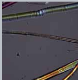
➍ Fibras del tejido original vistas al microscopio óptico / FOTO: LOURDES MARTÍN, IAPH
