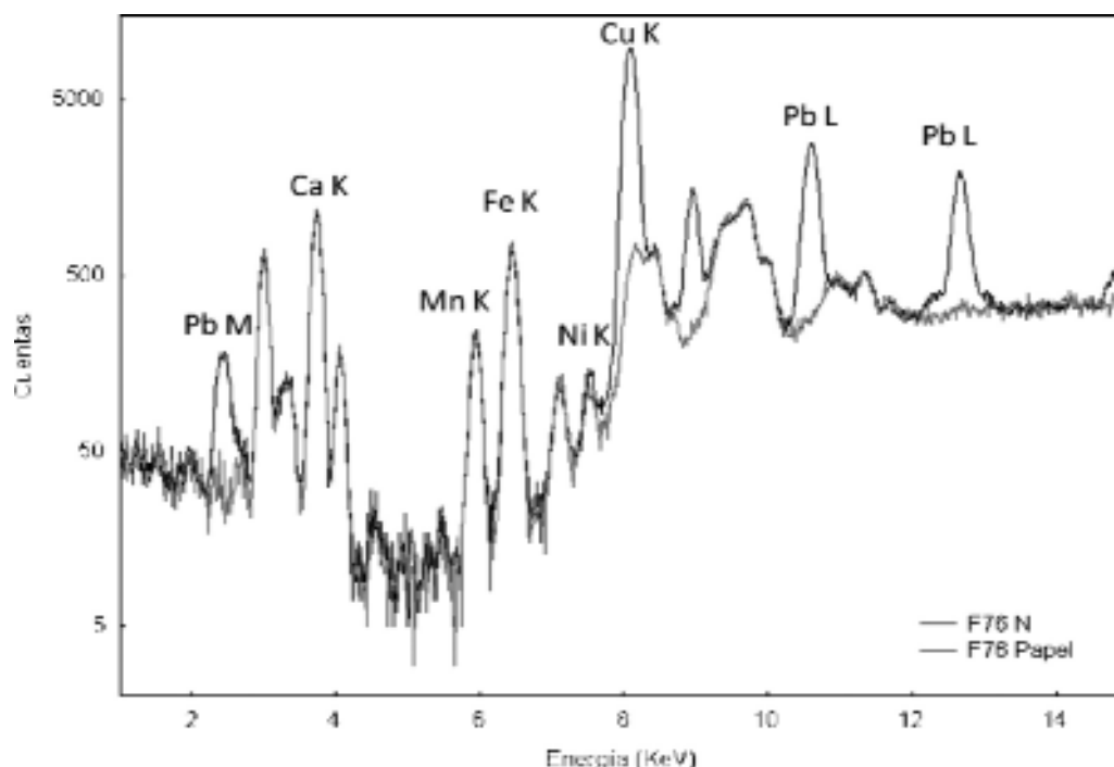
Figura 1. Espectros de la tinta negra (F76N) y del papel del Folio 76.
