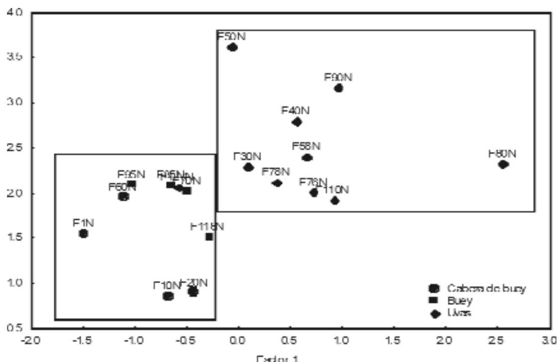
Figura 6. Representación del Factor 1 (Ti, Mn, y Fe del papel, frente la relación de áreas entre las líneas K del Cu y L del Pb, características de la tinta.
