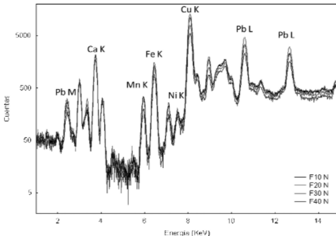
Figura 2. Espectros de caracteres tipográficos con tinta negra.
