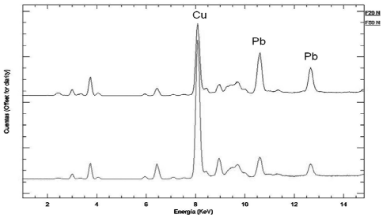
Figura 3. Variabilidad de los espectros de caracteres tipográficos con tinta negra.
