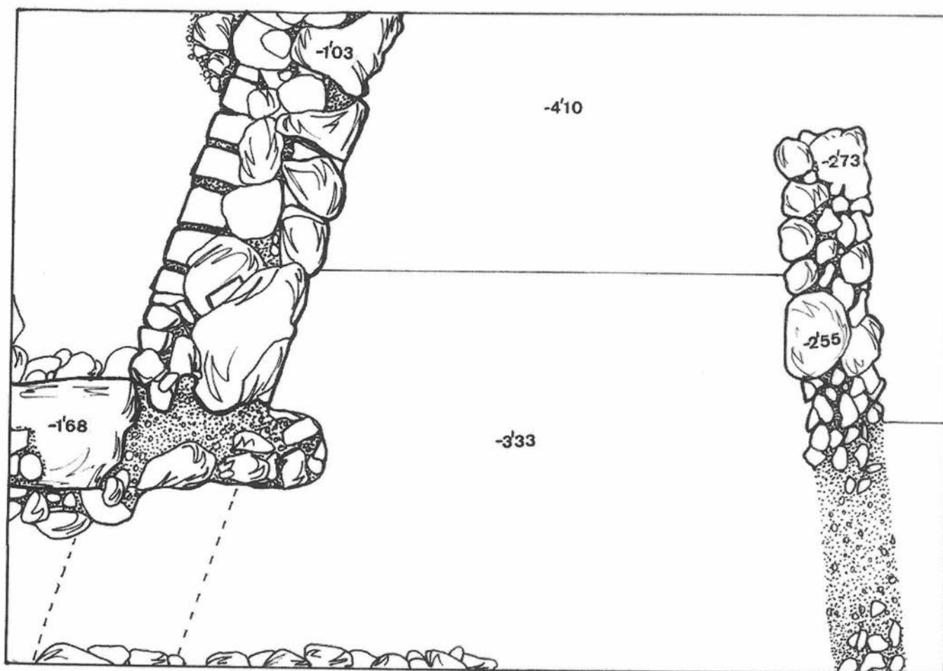
FIG. 5. Planta general del corte.
