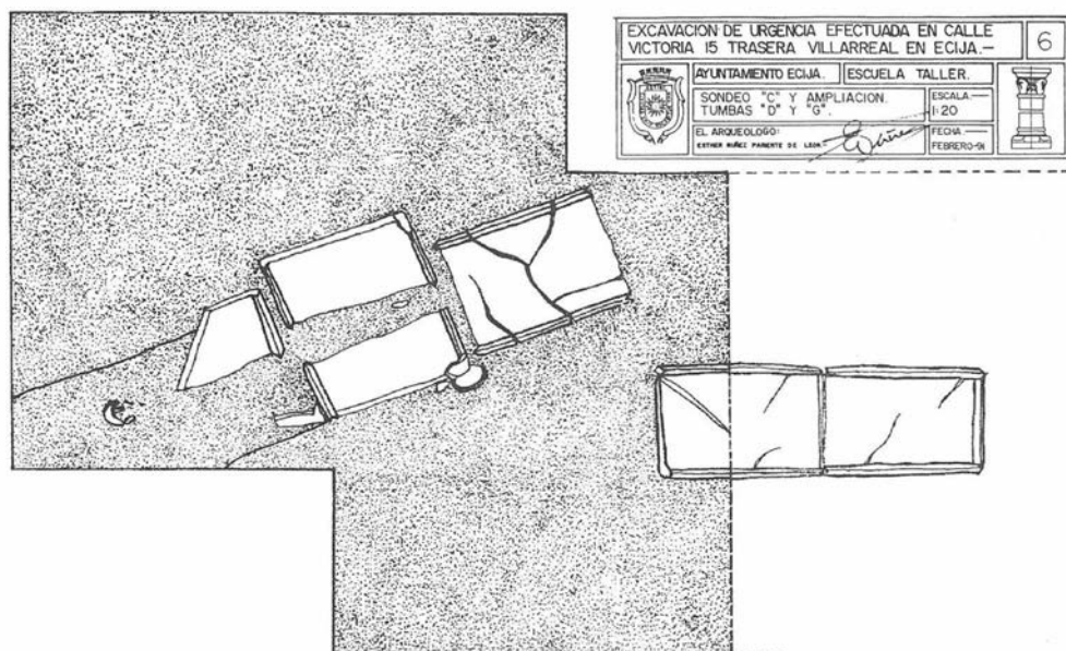
FIGURA 6. Planta de las Tumba "D" y "G".
