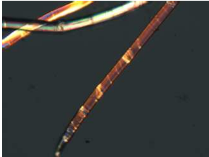
Fotomicrografía de la apariencia longitudinal de algunas fibras al microscopio óptico con luz transmitida (200X).
