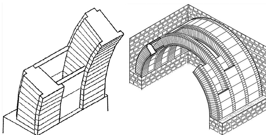
Fig. 15. Reconstrucción de la conexión entre dovelas y tejas en el método del "double-slab armchair voussoir vault" , en este caso con doble hilera de losas [Lancaster, 2015, fig. 101, detalle; Lancaster, 2015b, fig. 1.].
